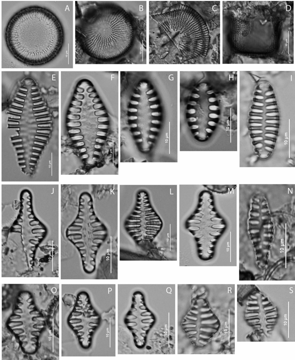
Fig. 9. Light microscope images (A–S): Ellerbeckia kochii (Pant.) Moiss. (A), Melosira undulata (Ehr.) Kütz. (B–D), Staurosirella sp. 1 (E–H), Staurosirella leptostauron var. dubia (Grun.) Edlund (I), Staurosirella leptostauron (Ehr.) Williams et Round (J–M, O–S), Staurosirella martyi (Hérib.) Morales et Manoylov (N).
